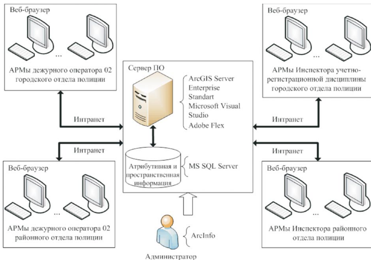
Рис. 2. Архитектура информационной системы экстренной службы «02»
