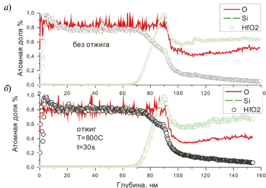
Рис. 5. Масс-спектр вторичных ионов (разрез подложки 200 мм): а – без отжига; б – с отжигом
