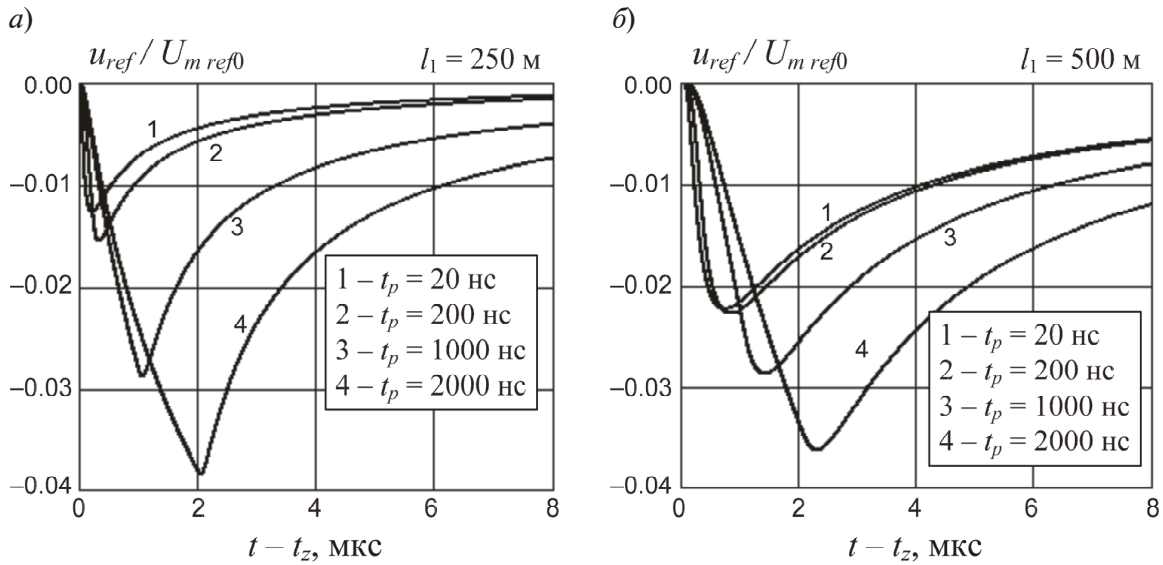
Рис. 6. Теоретически рассчитанные фрагменты рефлектограмм КЦ, состоящих из двух однородных участков, содержащие отраженные от стыка импульсы
