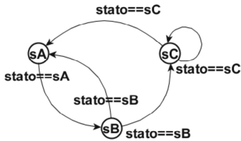
Рис. 3. Пример EFSM-модели
