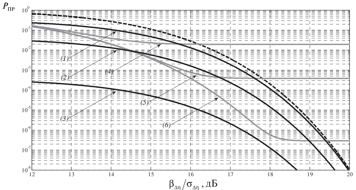
Рис. 14. Вероятности пропуска нарушения целостности НП при использовании результатов измерения двух углов на основе логического «ИЛИ» (кривые 1, 2 и 3), логического «И» (кривые 4, 5 и 6) и одного угла (пунктирная кривая) при P_{\text{лр}} = 10^{-5}
