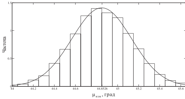
Рис. 6. Гистограмма распределения измеренного угла азимута, h^2 = 12 дБ
